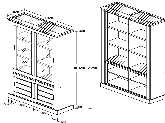
EVA MODEL : BC 70078G-S5V ITEM : GLASKAST / ARGENTIER / GLASS CABINET L 135 X D 46 X H 202cm
