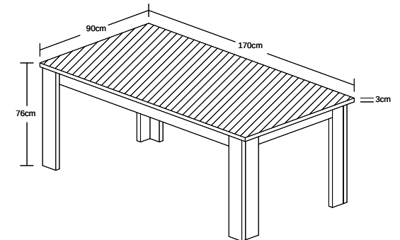
EMILY / EVA MODEL : DS 007-S5V ITEM : EETTAPEL / TABLE / DINING TABLE 170 L 170 X D 90 X H 76cm
