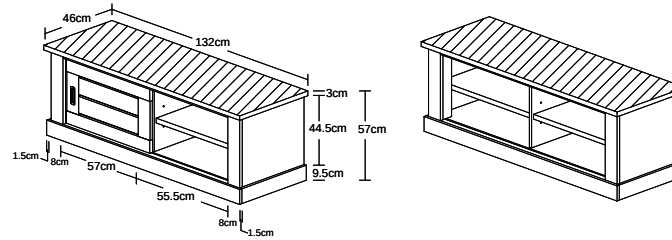
EVA MODEL : EC 60120-S5V ITEM : TV KAST / MEUBLE TV / TV CABINET L 132 X D 46 X H 57cm
