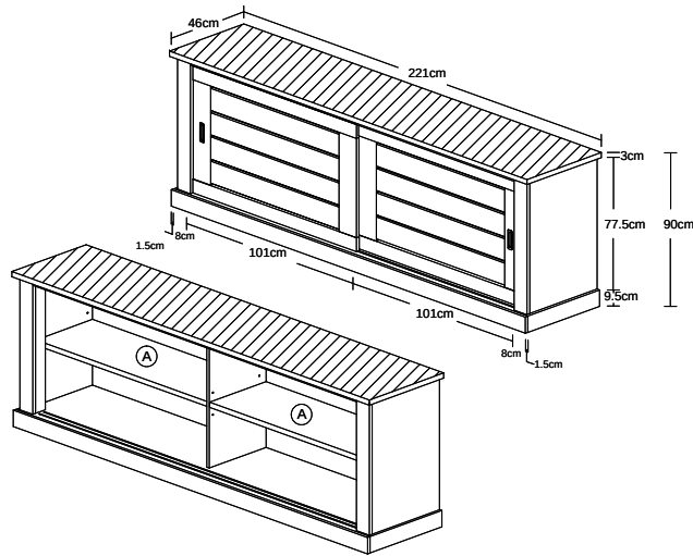
EVA MODEL : SB 190016-S5V ITEM : DRESSOIR 221 / SIDE BOARD L 221 X D 46 X H 90 cm
