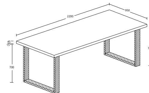
ESTRELLA MODEL : DS 032-S5V ITEM : DINING TABLE LEG: U METAL LEG L 220 X D 95 X H 76cm
