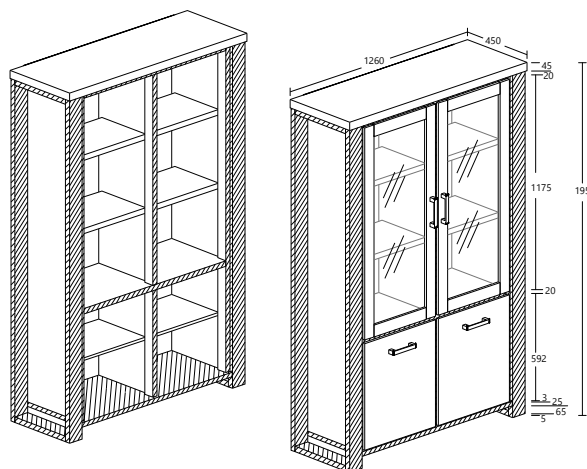
ESTRELLA MODEL : BC 70112G-S5V ITEM : GLASS CABINET L 126 X D 45 X H 195cm
