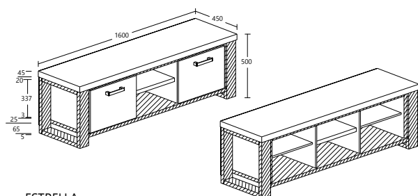
ESTRELLA MODEL : EC 60175-S5V ITEM : ENTERTAINMENT UNIT L 160 X D 45 X H 50cm
