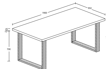
ESTRELLA MODEL : DS 028-S5V ITEM : DINING TABLE LEG: U METAL LEG L 190 X D 95 X H 76cm
