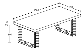
ESTRELLA MODEL : CT 15039-S5V ITEM : COFFEE TABLE LEG: U METAL LEG L 130 X D 65 X H 45cm
