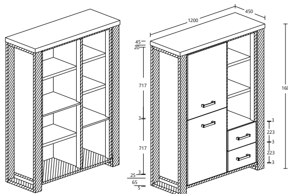
ESTRELLA MODEL : BC 70113-S5V ITEM : BAR L 120 X D 45 X H 160cm
