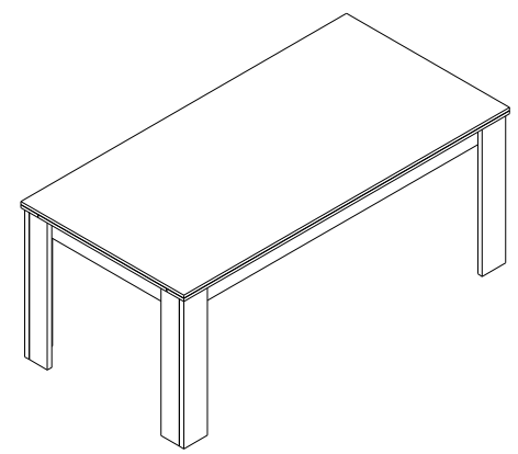
ESTHER Model: DN DT 660 107-IO Item: Eettafel / Table / Dining Table 180 L180 x D 90 x H 75cm
