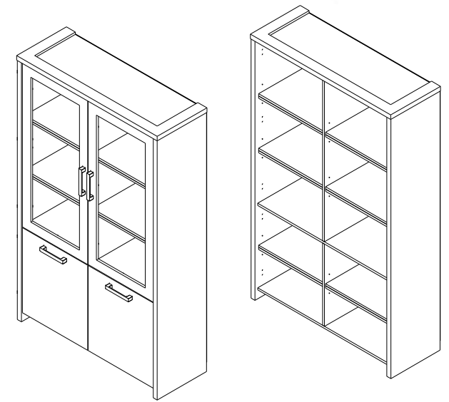
ESTHER Model: DN STC 201 635-IO Item: Glaskast / Argentier / Glass Cabinet L110 x D 39 x H 180cm
