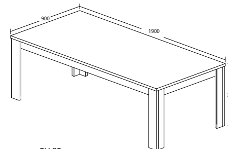
ELVIS MODEL : DS 020-S5V ITEM : EETTAfel / TABLE 190 / DINING TABLE 190 L 190 X D 90 X H76cm
