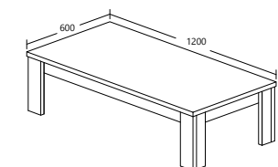
ELVIS MODEL : CT 15035-S5V ITEM : SALONTAFEL / TABLE BASSE 120 / SOFA TABLE 120 L 120 X D 60 X H40cm
