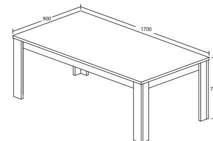
ELVIS MODEL : DS 019-S5V ITEM : EETTAfel / TABLE 170 / DINING TABLE 170 L 170 X D 90 X H76cm
