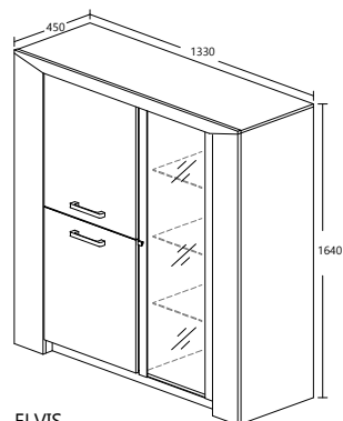
ELVIS MODEL : BC 70097-S5V ITEM : GLASKAST / ARGENTIER / GLASS CABINET L 133 X D 45 X H164cm
