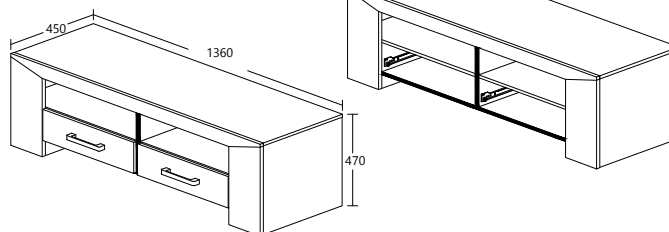
ELVIS MODEL : EC 60149-S5V ITEM : TV KAST / MEUBLE TV / TV CABINET L 136 X D 45 X H47cm
