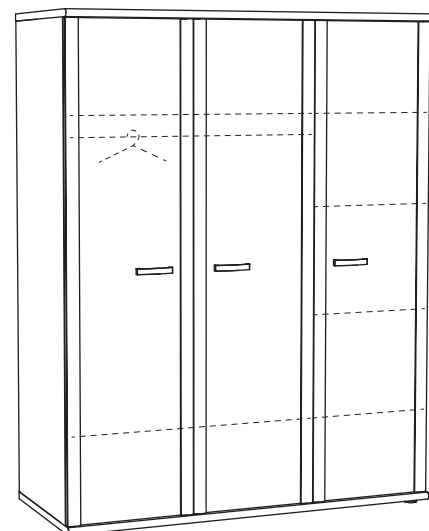
K3 150 x 194 x 64 cm
