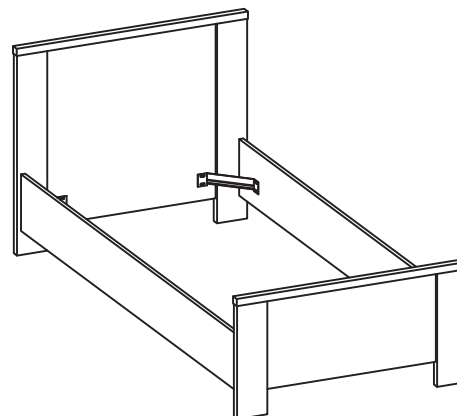
Item : BED 90 Model : DN BED 3659 L2064 x W995 x H860mm
