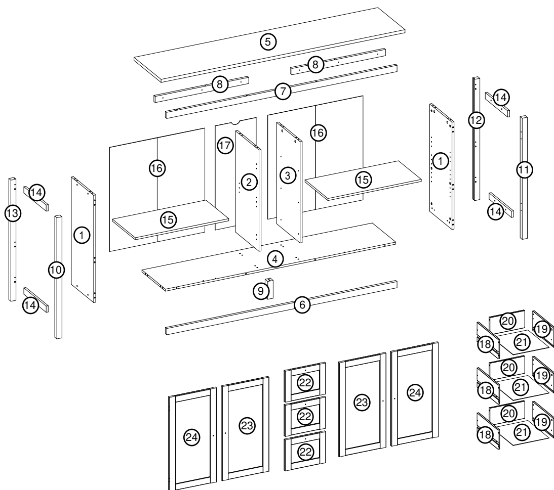
Dimensions / Abmessung in mm/
