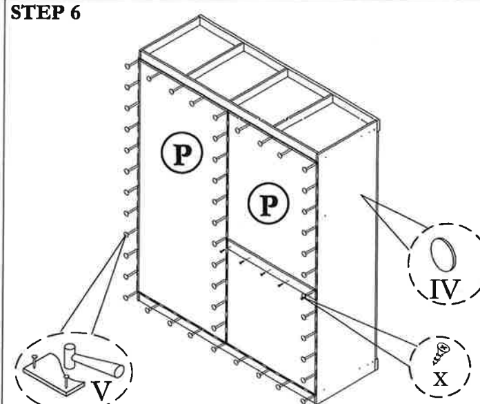
STEP 6
