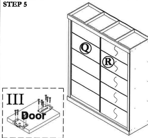
STEP 5
